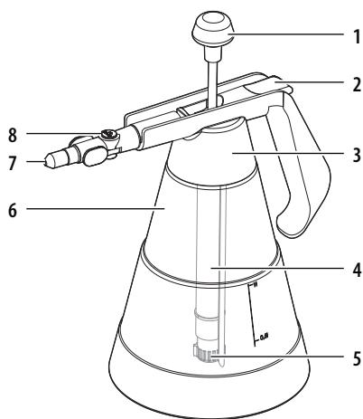
Fig. 1: Special-tryksprøjten
