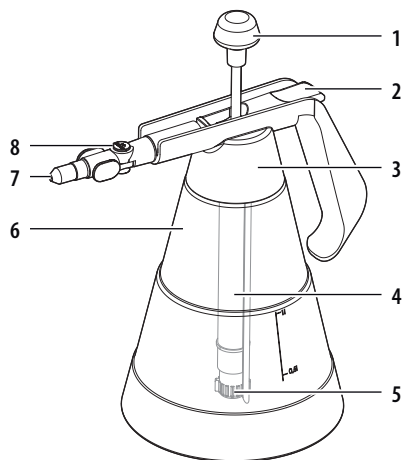
Fig. 1: Componentes del pulverizador a presión especial
